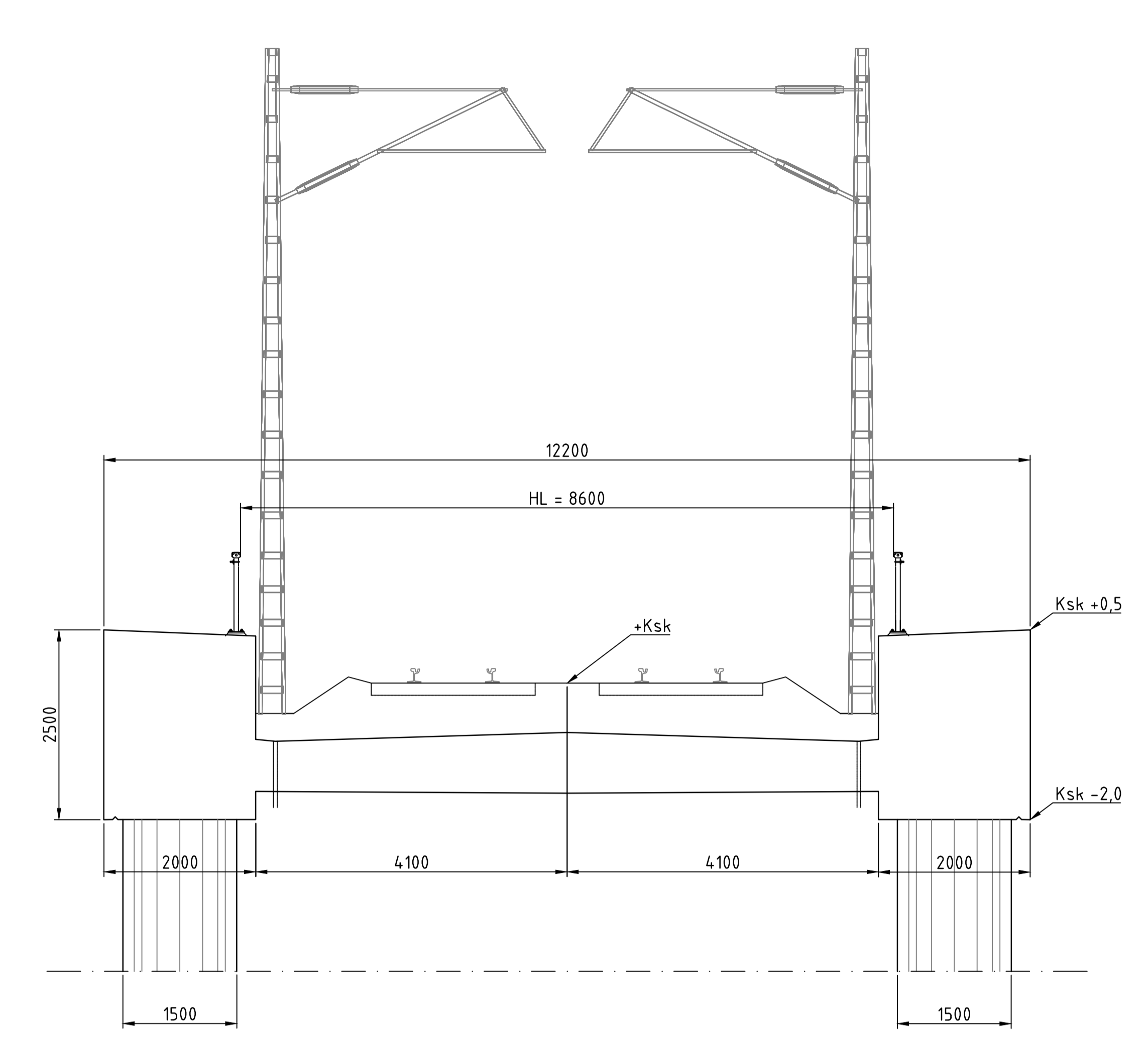
B-B 1:50
